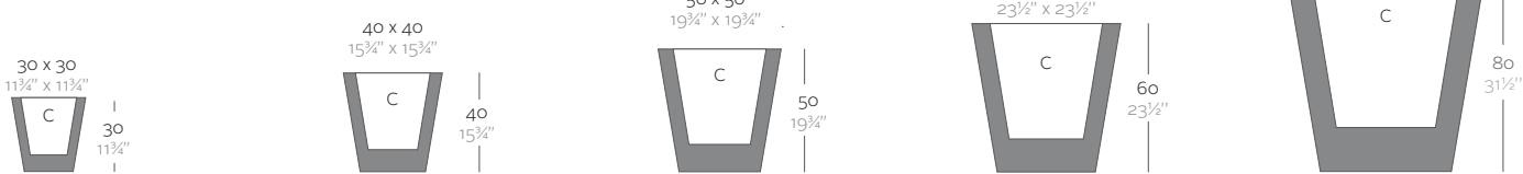
Squared Cone 11 3/4" Cono Cuadrado 30 cm Squared Cone 15 3/4" Cono Cuadrado 40 cm Squared Cone 19 3/4" Cono Cuadrado 50 cm Squared Cone 23 1/2" Cono Cuadrado 60 cm Squared Cone 31 1/2" Cono Cuadrado 80 cm
