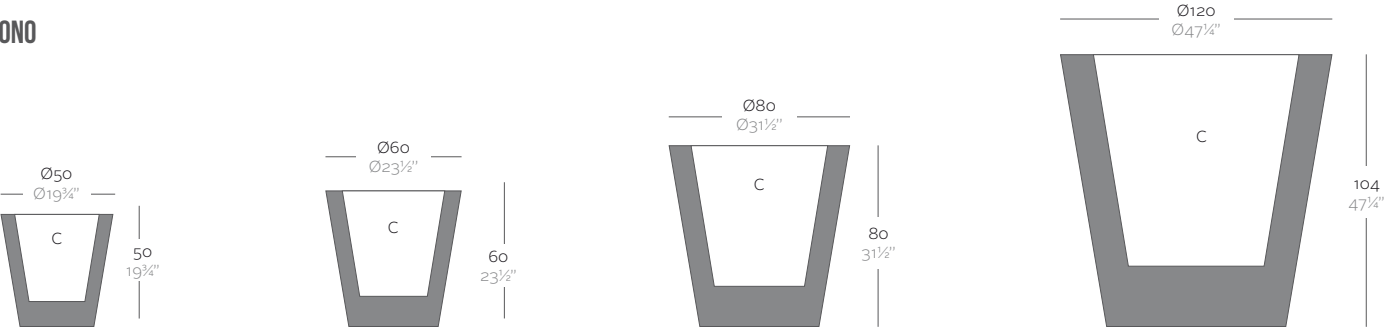
Cono Ø19½" Cono Ø50 cm Cono Ø23½" Cono Ø60 cm Cono Ø31½" Cono Ø80 cm Cono Ø47¼" Cono Ø120 cm
