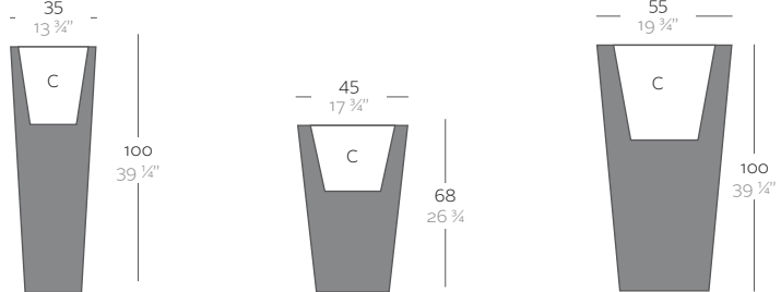
Square High Cone 13 3/4" Cono Cuadrado Alto 35 cm Square High Cone 17 3/4" Cono Cuadrado Alto 45 cm Square High Cone 23 1/2" Cono Cuadrado Alto 55 cm
